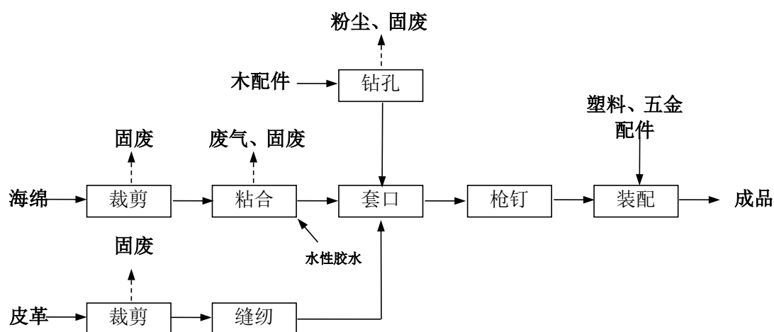
图 2-2 原有项目家具及转椅生产工艺流程图示（噪声伴随整个生产过程）
