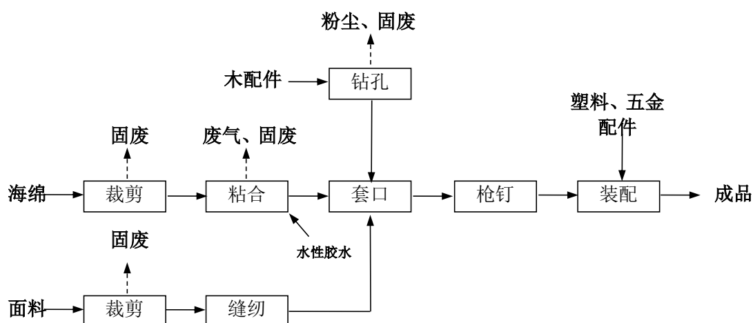
图 2-2 坐具生产工艺流程图示（噪声伴随整个生产过程）
