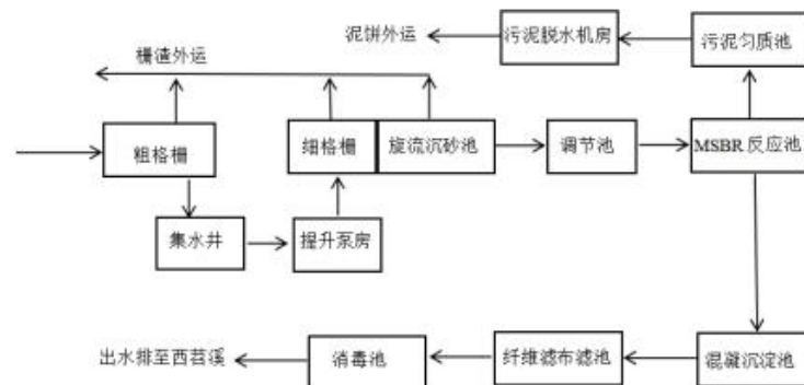
图 4-2 安吉净源污水处理有限公司城北污水处理厂三期处理工艺图
