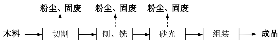
图 2-3 原有项目转椅配件生产工艺流程图示（噪声伴随整个生产过程）
