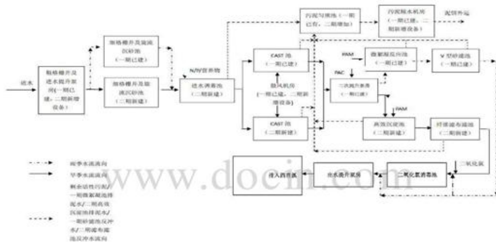
图 4-1 安吉净源污水处理有限公司城北污水处理厂一期、二期处理工艺图
