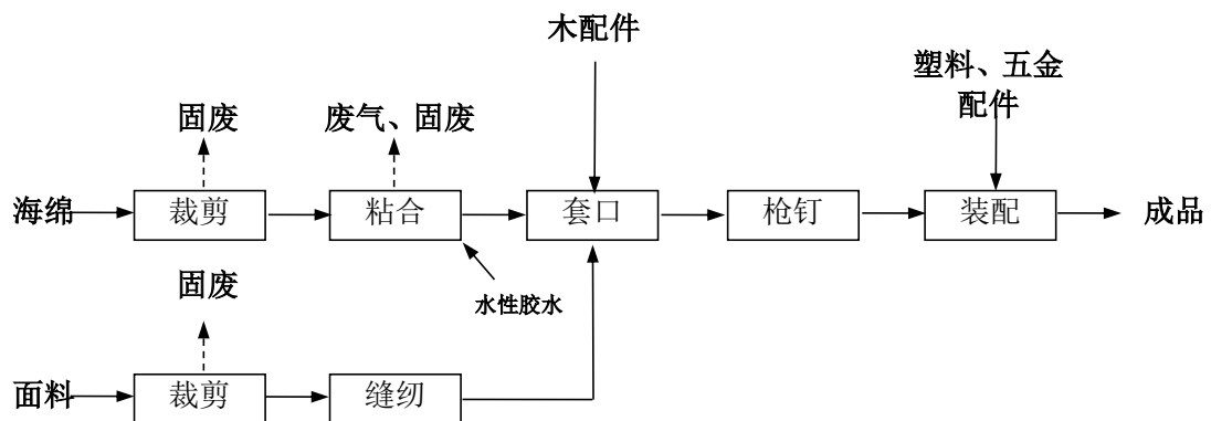
图 2-2 中高档休闲椅生产工艺流程图示（噪声伴随整个生产过程）
