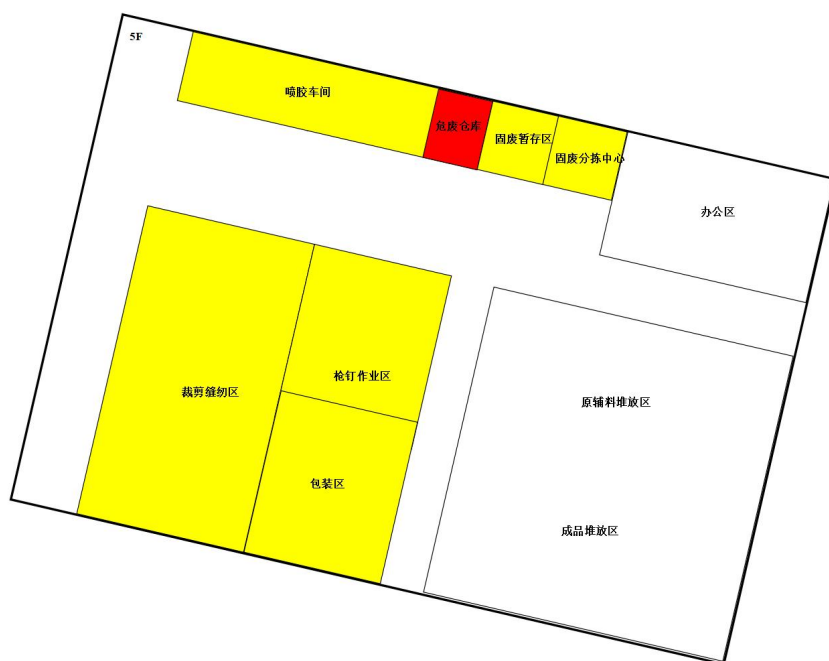
图 4-3 本项目分区防渗图
