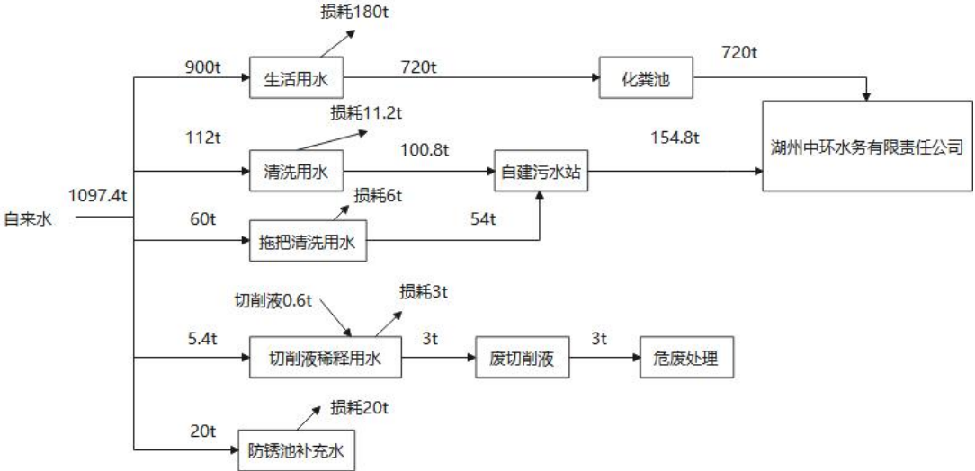
图 2-3 水平衡图
