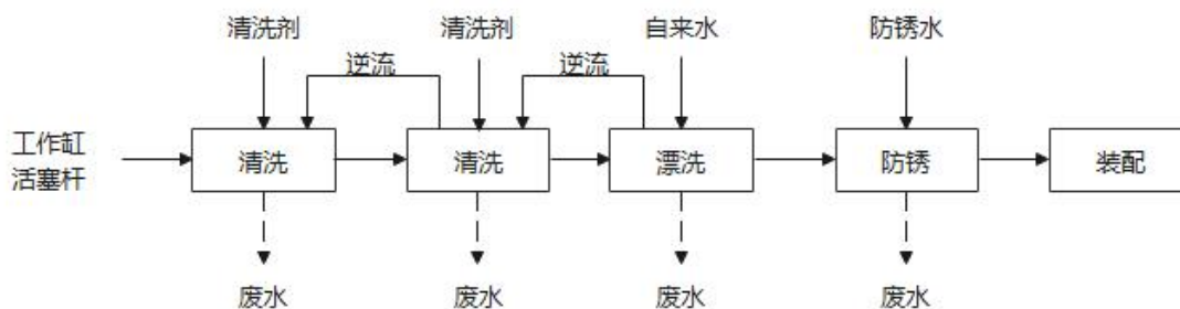
图2-7 超声波清洗机工作图
