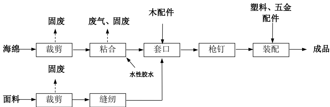
图 2-2 智能办公系统家具生产工艺流程图示（噪声伴随整个生产过程）
