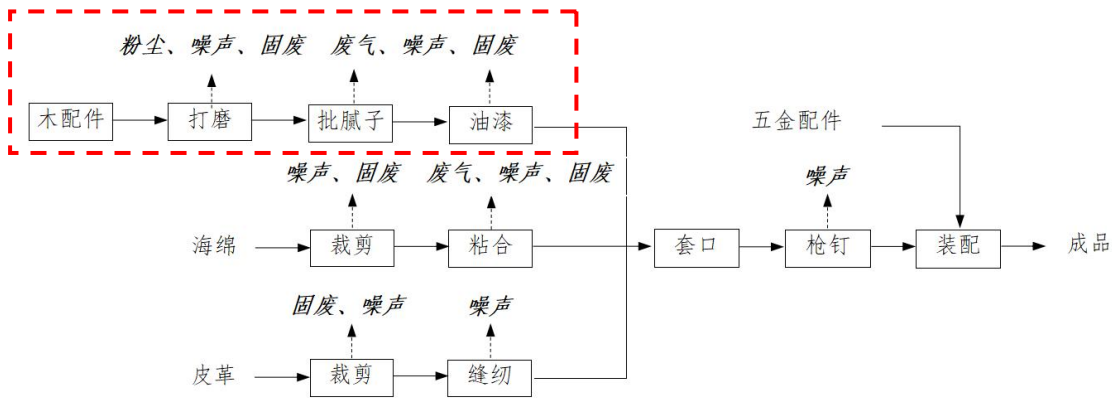
图 2-3 原有项目家具生产工艺流程图示（噪声伴随整个生产过程）
