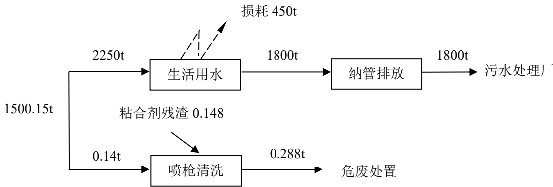
图 2-1 本项目实施后水平衡图 (t/a)
