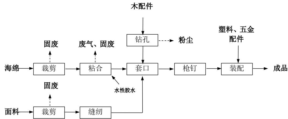
图 2-3 中高档转椅生产工艺流程图示（噪声伴随整个生产过程）
