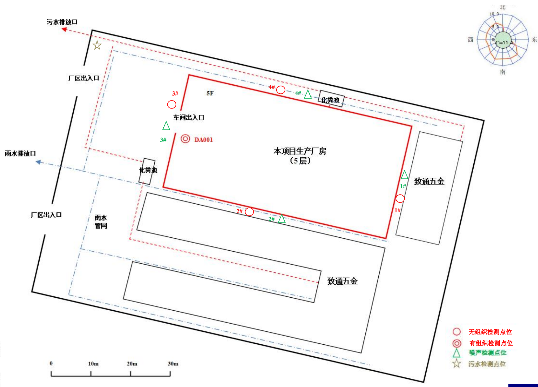
● 附图 5 建设项目监测点位示意图
